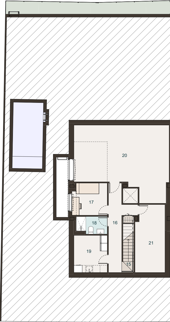
PLANTA SÓTANO
