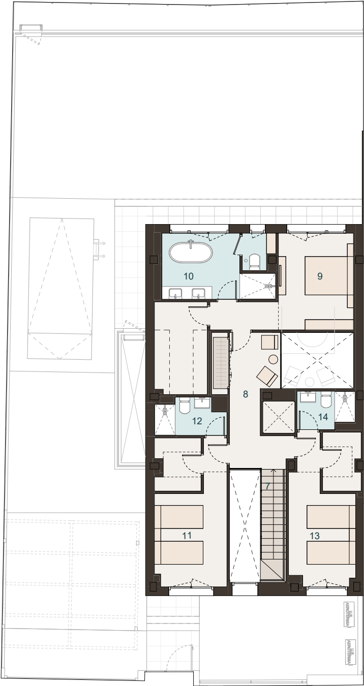
PLANTA PRIMERA
