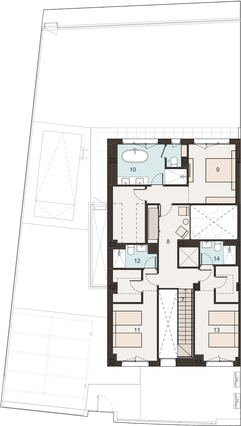
PLANTA PRIMERA
