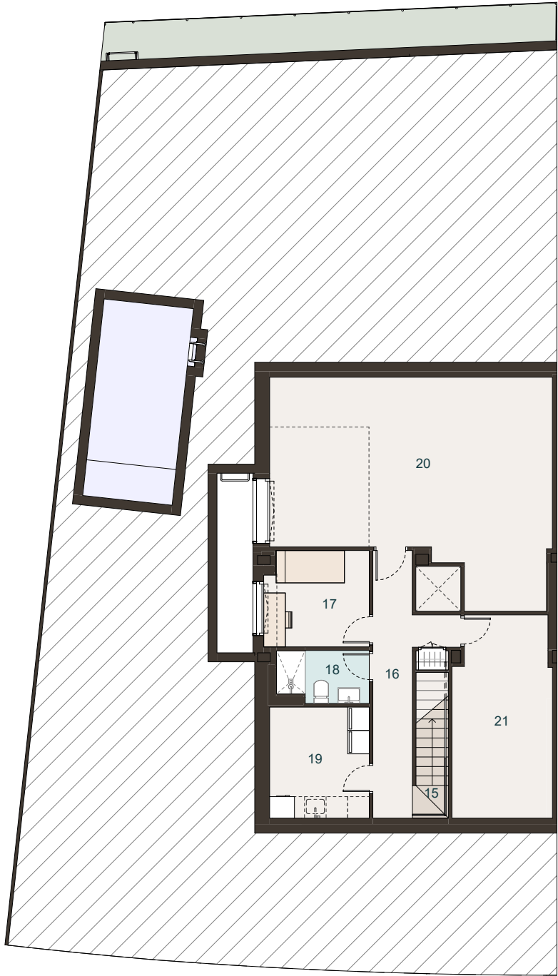
PLANTA SÓTANO
