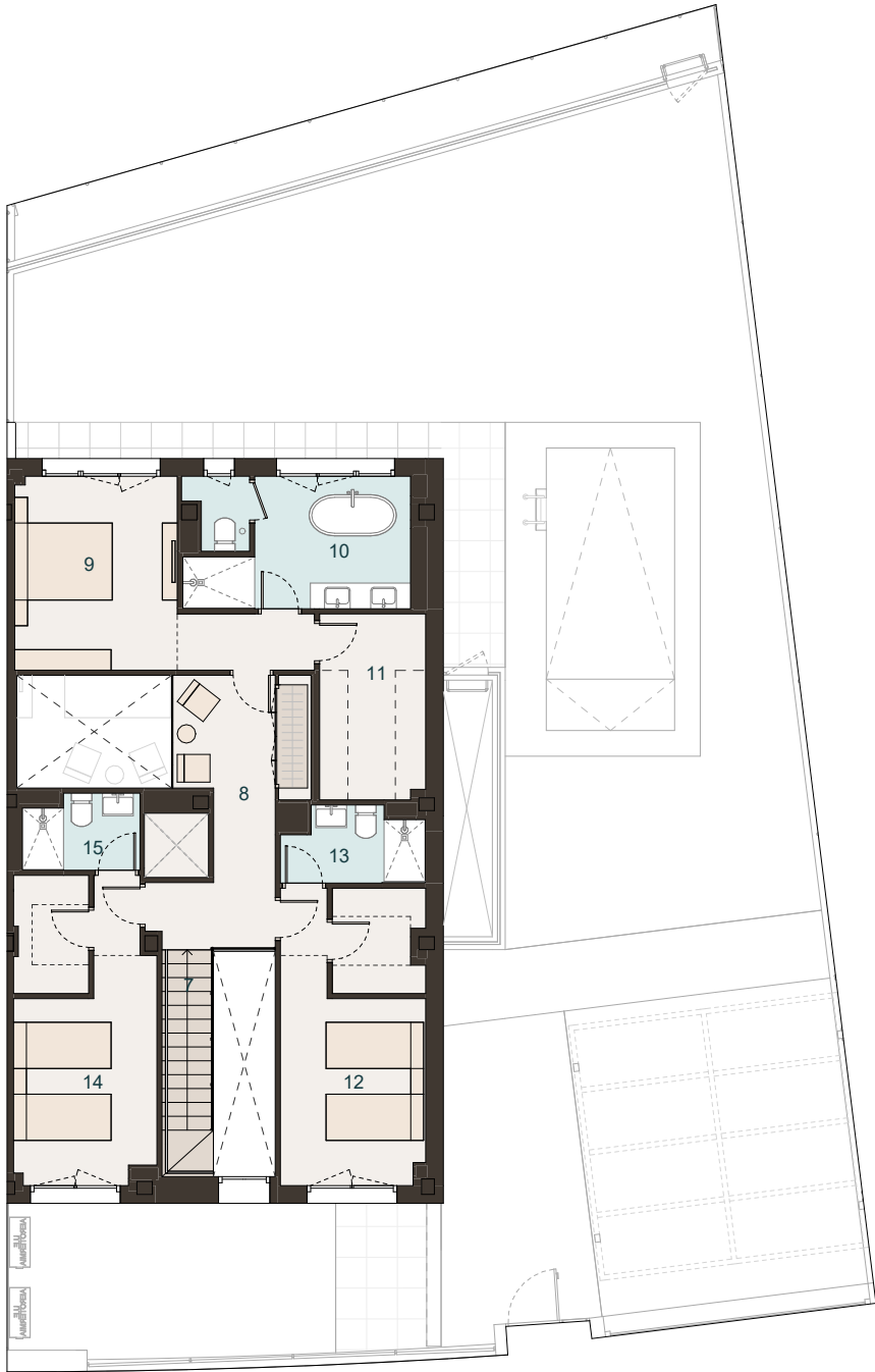
PLANTA PRIMERA
