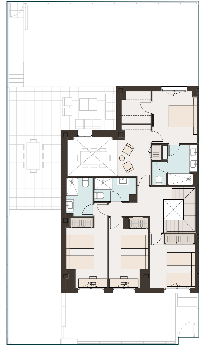
PLANTA PRIMERA
