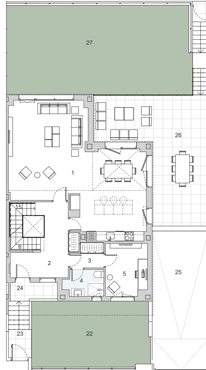
PLANTA BAJA
